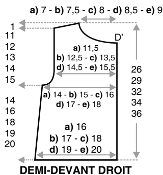
DEMI-DEVANT DROIT
